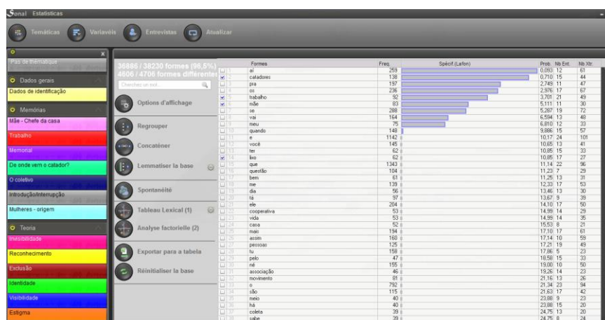
Figura 33 – Análise léxica
